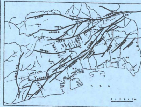
神戸の断層
