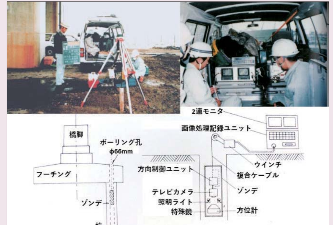
写真7 ボアホールカメラでの基礎杭調査状況
