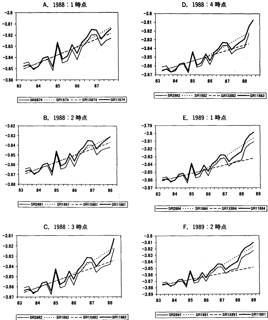
図3. ソロー残差の推計値, 屈折トレンド, 固定トレンド
