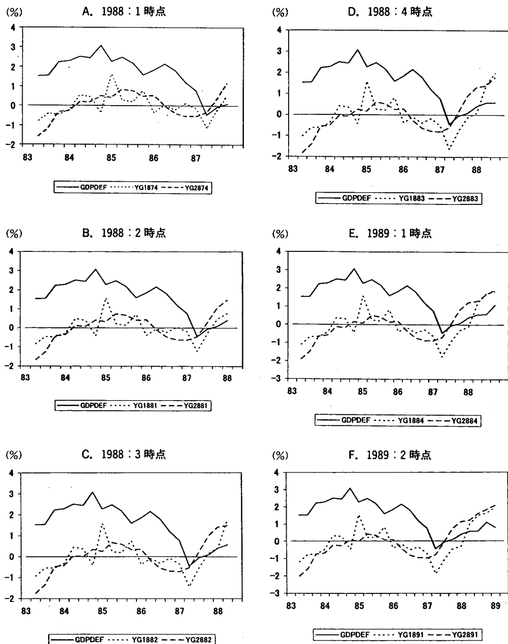
図4. GDP デフレーター・インフレ率と GDP ギャップ —従来型 vs 修正型—
