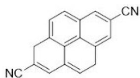
2,7-dicyanopyrene
