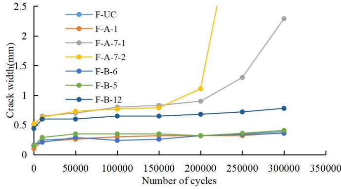
Fig. 5.8 Crack width
