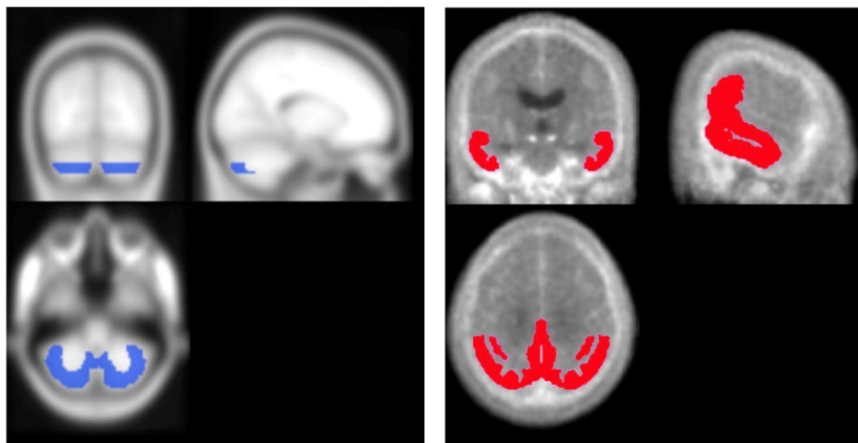
Fig. 2 Reference VOIs for the CenTauR scale. Blue : cerebellar VOI, red : tau deposition target VOI
