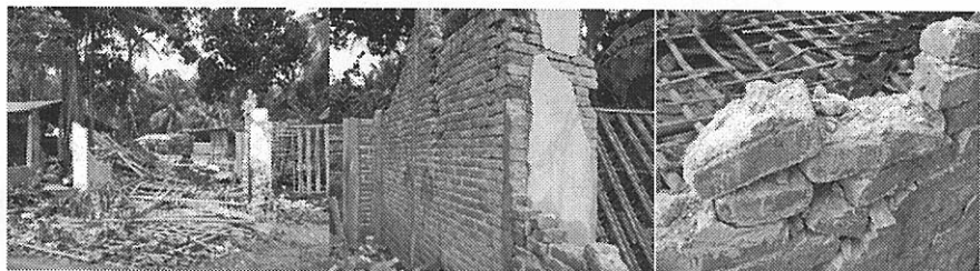
写真-15 倒壊家屋の構造 (Pandak)
