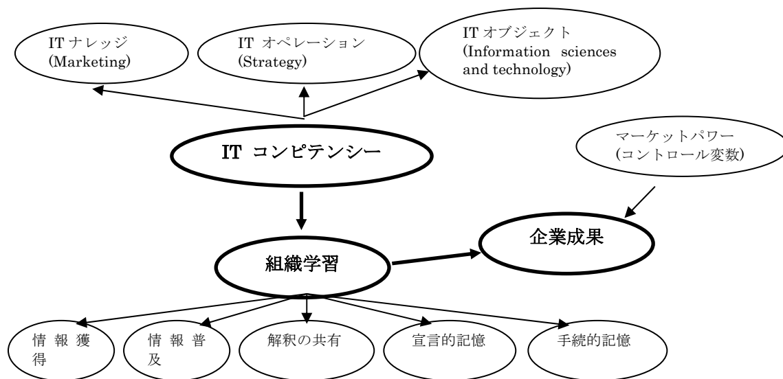
図 Tippins and Sohi (2003) による分析モデル 誤差および測定方程式については省略
