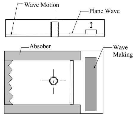
Fig.4 Ripple-Tank
