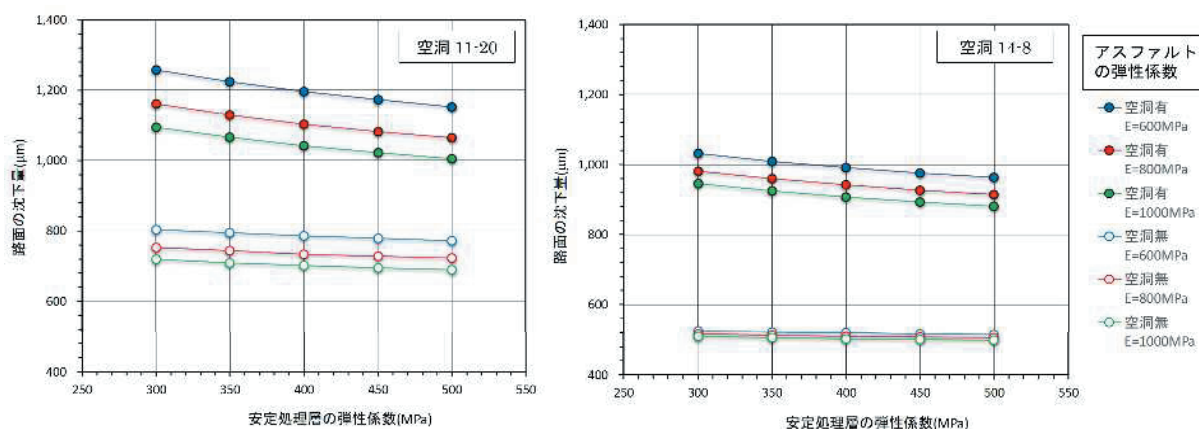
図 10 たわみ量( D_0 )とアスファルト及び安定処理層の弾性係数の関係
