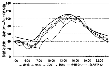
図9 総括対流熱伝達率の時刻別平均値（鉄塔） 図10 総括対流熱伝達率の標準偏差（鉄塔）
