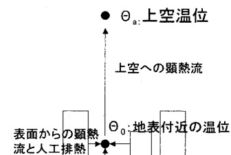
図3 接地境界層モデルのイメージ
