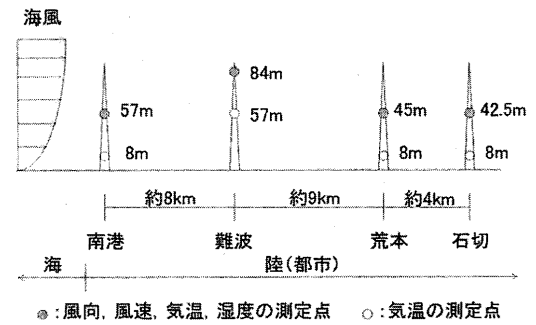
図2 鉄塔を用いた上空気象測定の概要
