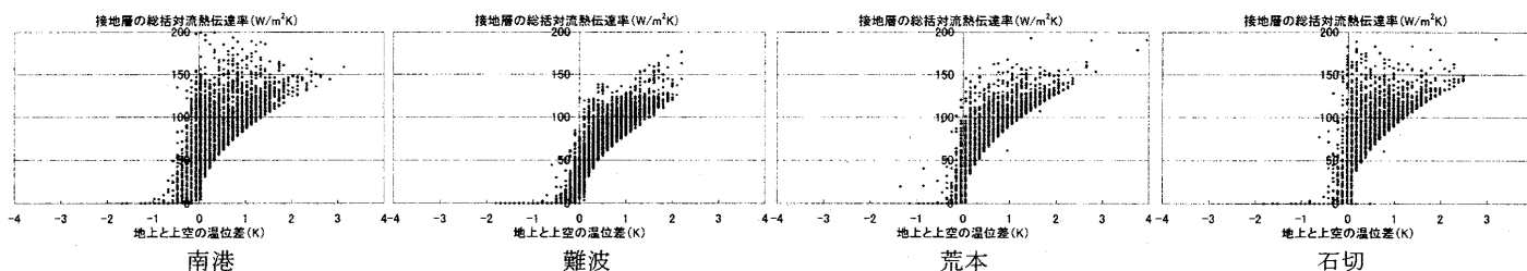
図5 鉄塔の観測データを用いた地上と上空の温位差と接地層の総括対流熱伝達率の関係（2006年8月1日～31日）
