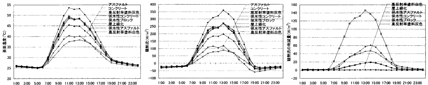
図11 表面温度、顕熱流、顕熱流の削減量の計算結果(2006年8月1日～8月31日の時刻別平均)
