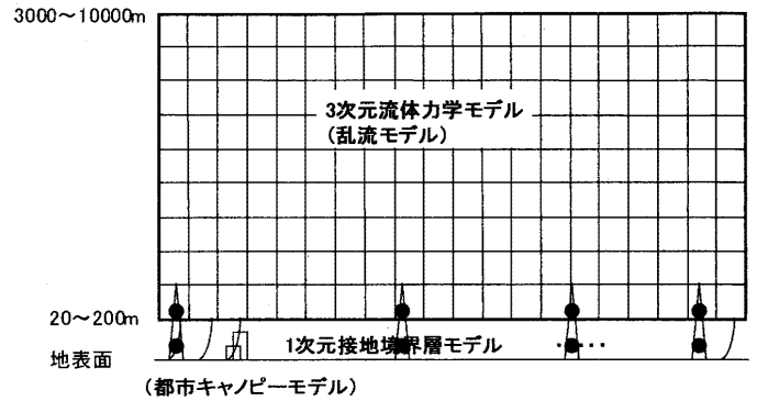
図1 一般的なメソスケールの気象シミュレーションモデルの構成のイメージ及び鉄塔での観測のイメージ
