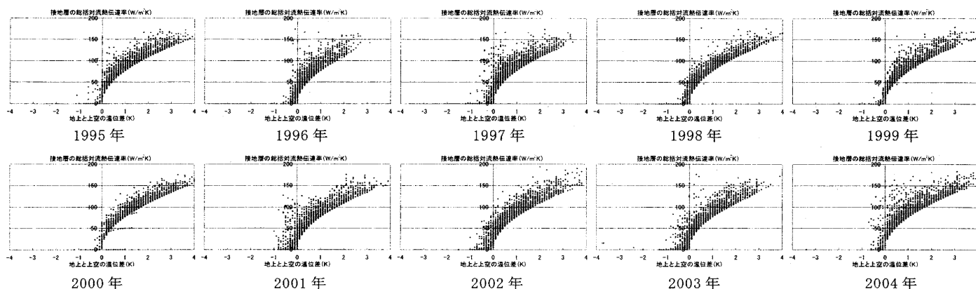
図4 大阪タワーの観測データを用いた地上と上空の温位差と接地層の総括対流熱伝達率の関係（各年7月1日～9月30日）
