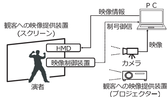
図 12 システム構成
