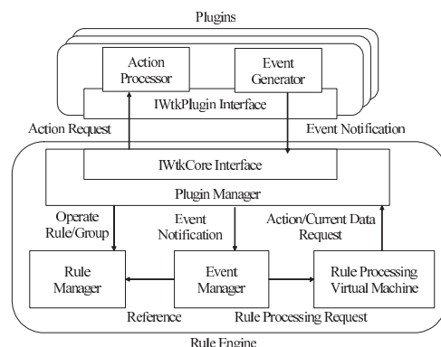
図 5 ルール処理エンジンの構成
