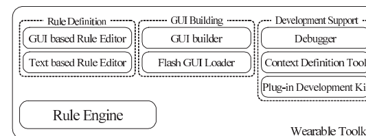
図 2 Wearable Toolkit の構成
