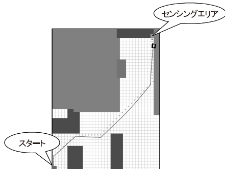
図 17 実装結果 (提案アルゴリズム) Fig. 17 Mounting result by the proposed algorithm.
