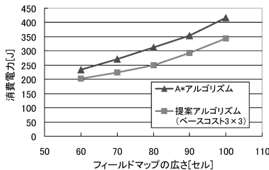
図 12 フィールドマップの広さ変化による目的地までの消費電力 (戦車型ノード)
