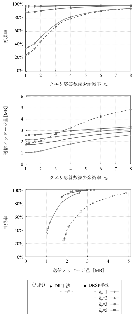
図 5 r_m の変化に対する再現率およびメッセージ量、およびメッセージ量の変化に対する再現率
