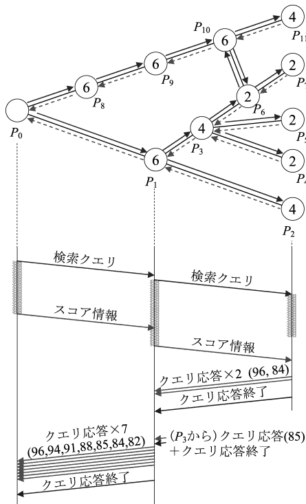
図 3 DRSP 手法における検索手順と各ピアが返信するクエリ応答の例
