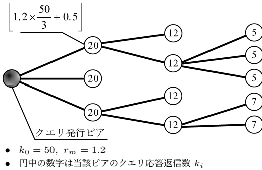
図2 DR 手法におけるクエリ応答返信数
