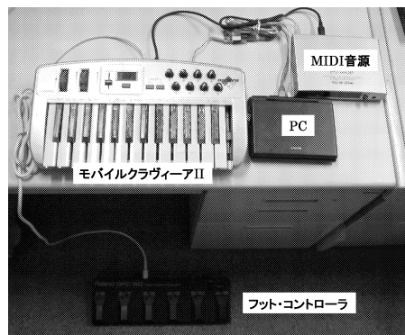
図 4 システム構成
