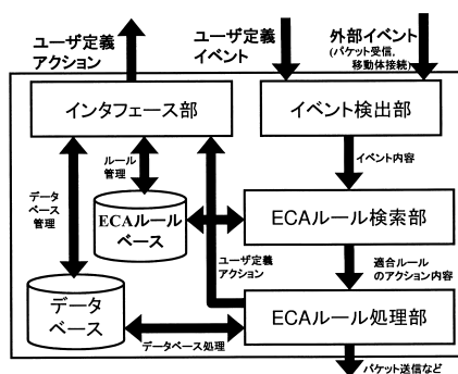
図5 AMDSモジュールのシステム構成
