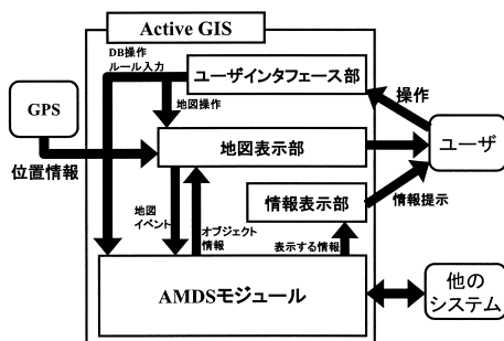
図3 ActiveGISのシステム構成
