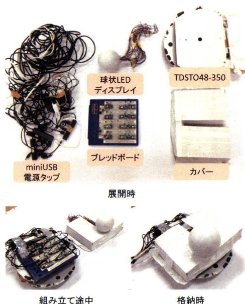
図3 球状LEDディスプレイと移動ロボットの連結
