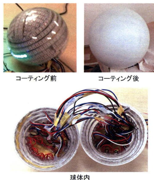
図4 球状LEDディスプレイの外観
