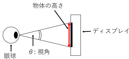
図 2 logMAR の定義
