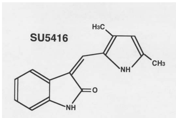
FIG. 1. SU5416.
