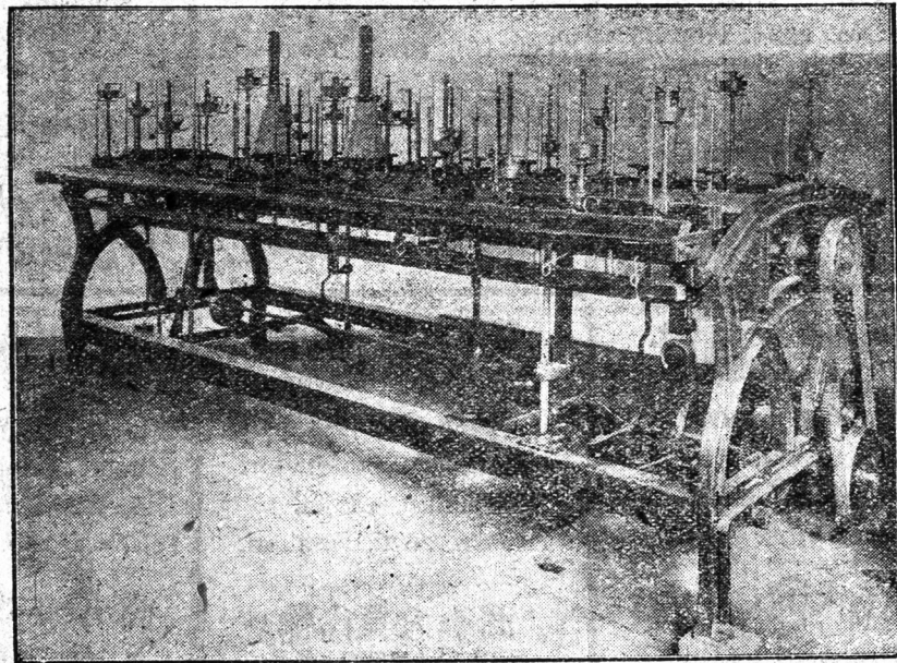
械機繰絲一ダンイワ式木鈴
